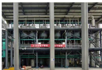
黄冈TCL环境科技有限公司 物化废水 4T/H三效蒸发器 2套
